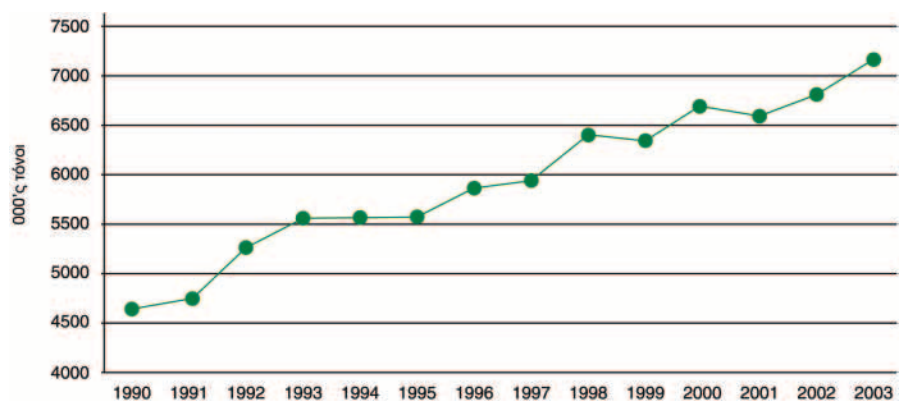
Αέριες Εκπομπές Διοξειδίου του Άνθρακα (CO2), 1990 - 2003
