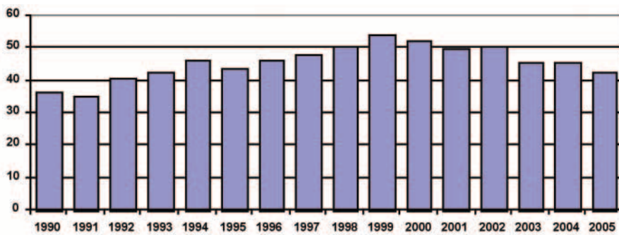
Συνολικές Ετήσιες Εκπομπές Διοξειδίου του Θείου (SO2) κατά την Περίοδο 1990 - 2005
