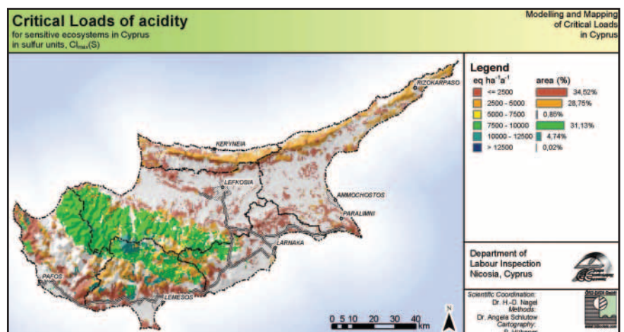
Χάρτης Κρίσιμων Περιβαλλοντικών Φορτίων Οξίνισης στην Κύπρο
