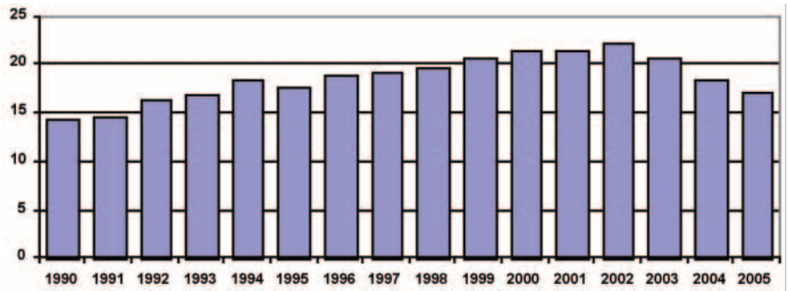
Συνολικές Ετήσιες Εκπομπές Οξειδίων του Αζώτου (NOx) κατά την Περίοδο 1990 - 2005
